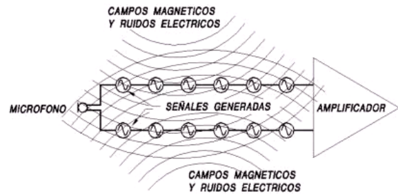
Fig. 5 Efecto de los campos magnéticos y eléctricos sobre un conductor.
