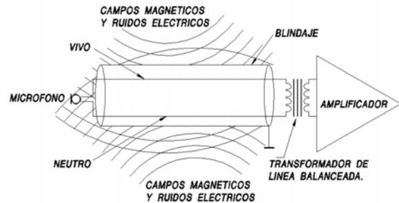
Fig. 8 Conexión Balanceada.
