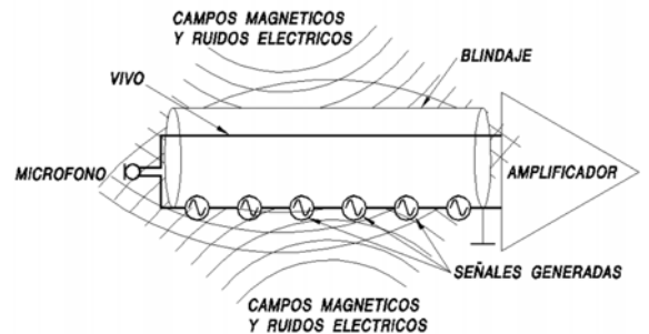
Fig. 6 Conexión con cable blindado sencillo.
