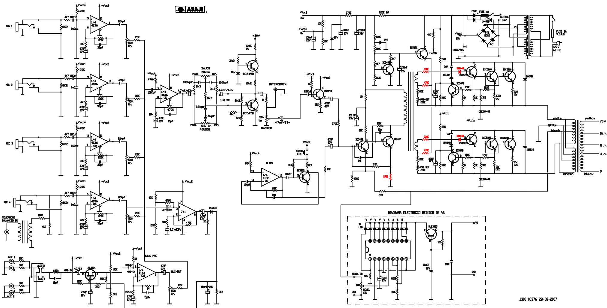
DIAGRAMA ELECTRICO DEL AMPLIFICADOR MEZCLADOR DE AUDIO MODELO 1094
